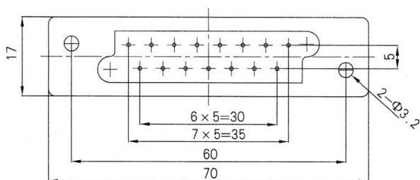
Receptacle (ZJA15K, ZJA15K-01)
