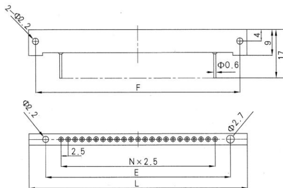
Receptacle (ZJA23K, ZJA29K)
