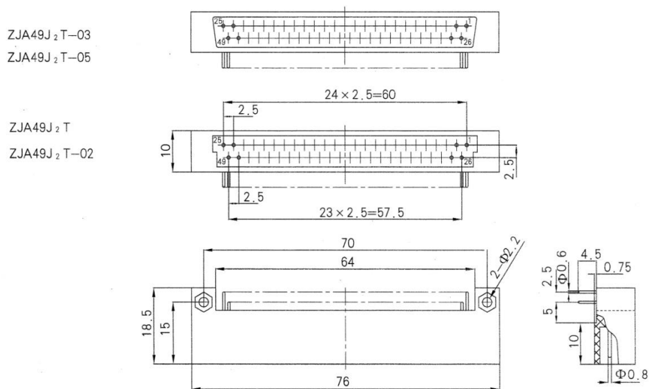
Plug (ZJA49J 2 T, ZJA49J 2 T-02, ZJA49J 2 T-03, ZJA49J 2 T-05)
