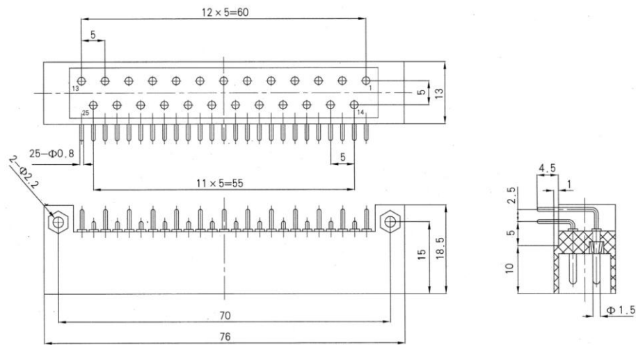
Plug (ZJA25J 2 T, ZJA25J 2 T-01, ZJA25J 2 T-02, ZJA25J 2 T-04, ZJA25J 2 T-05)
