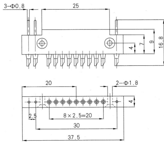
Receptacle (ZJA12-01)
