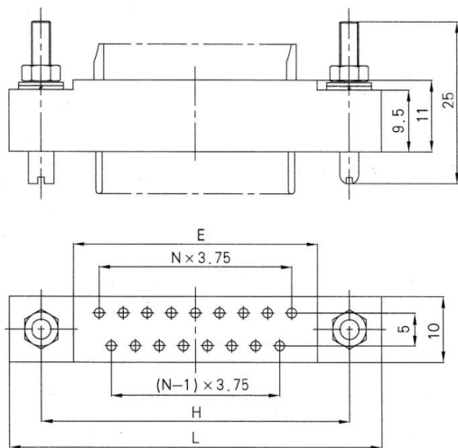
Plug (ZJA17J 1 T, ZJA27J 1 T, ZJA33J 1 T)
