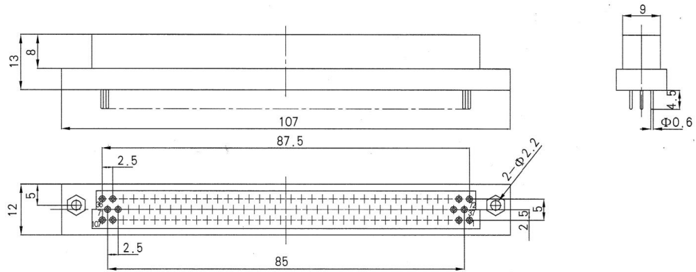
Receptacle (ZJA120J 2 T)
