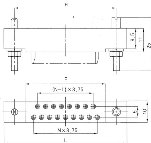
Receptacle (ZJA17K, ZJA27K, ZJA33K)
