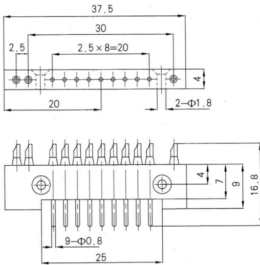
Plug (ZJA12-01T)
