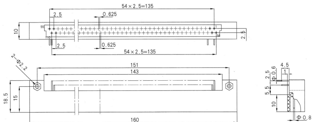
Plug (ZJA110J 2 T, ZJA110J 2 T-01, ZJA110J 2 T-02)
