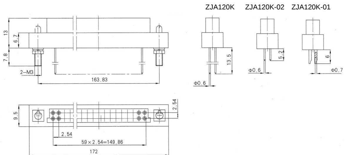
Receptacle (ZJA120K, ZJA120K-01, ZJA120K-02)
