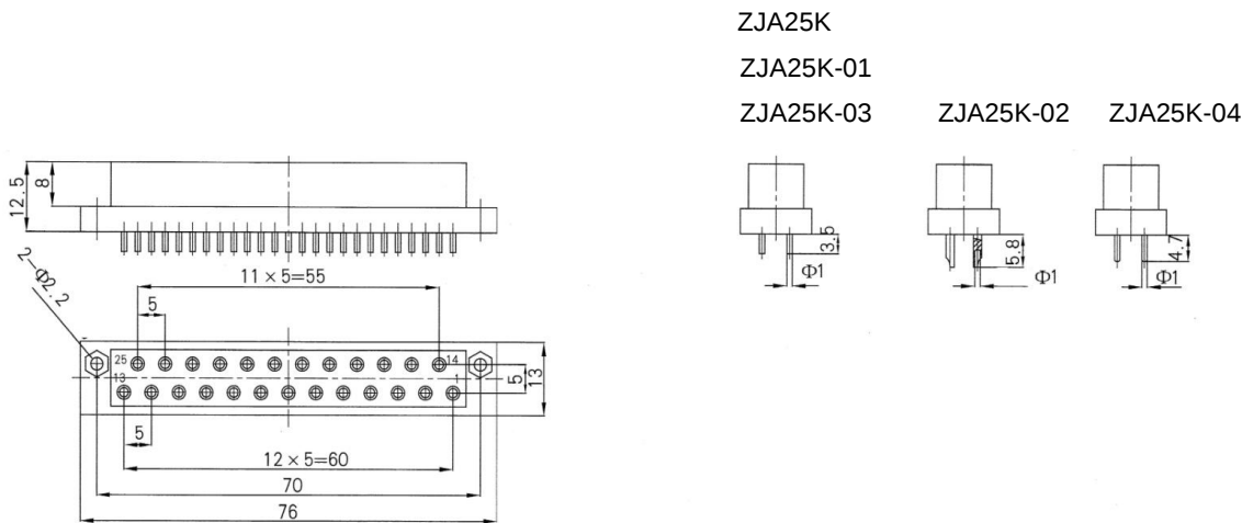
Receptacle (ZJA25K, ZJA25K-01, ZJA25K-02, ZJA25K-03, ZJA25K-04)
