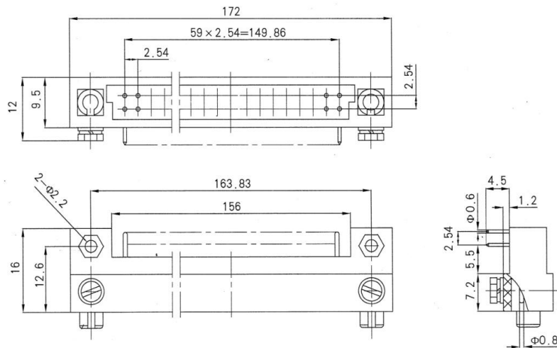
Plug (ZJA120J 2 T)
