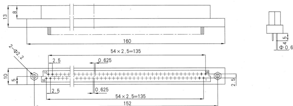
Receptacle (ZJA110K, ZJA110K-01, ZJA110K-03)
