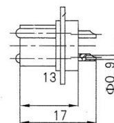
ZJA15K
