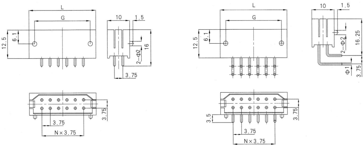
Receptacle (ZJA12J 1 , ZJA20J 1 )
