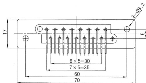
Plug (ZJA15J 2 T)
